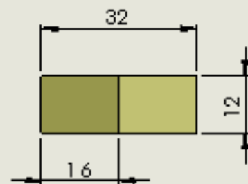
End Elevation
